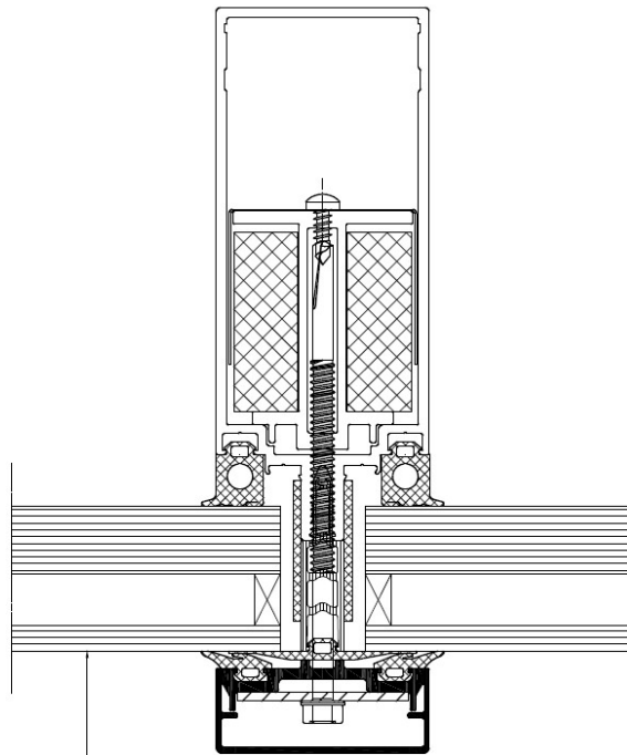
① CONTRAFLAM 30 CLIMAPLUS (minimum edge cover = 15 mm vertical edges 15 mm top edge 13 mm bottom edge)
