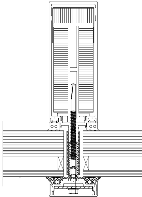
① CONTRAFLAM 60-3 CLIMAPLUS (minimum edge cover = 15 mm vertical edges 15 mm top edge 13 mm bottom edge)
